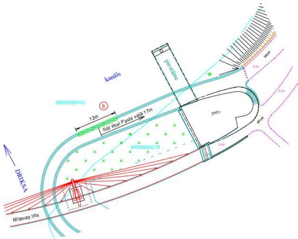
Stāvvietas izvietojuma shēma
