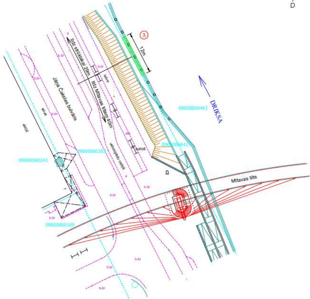
Stāvvietas izvietojuma shēma
