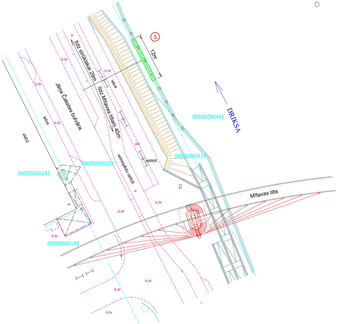
Stāvvietas izvietojuma shēma
